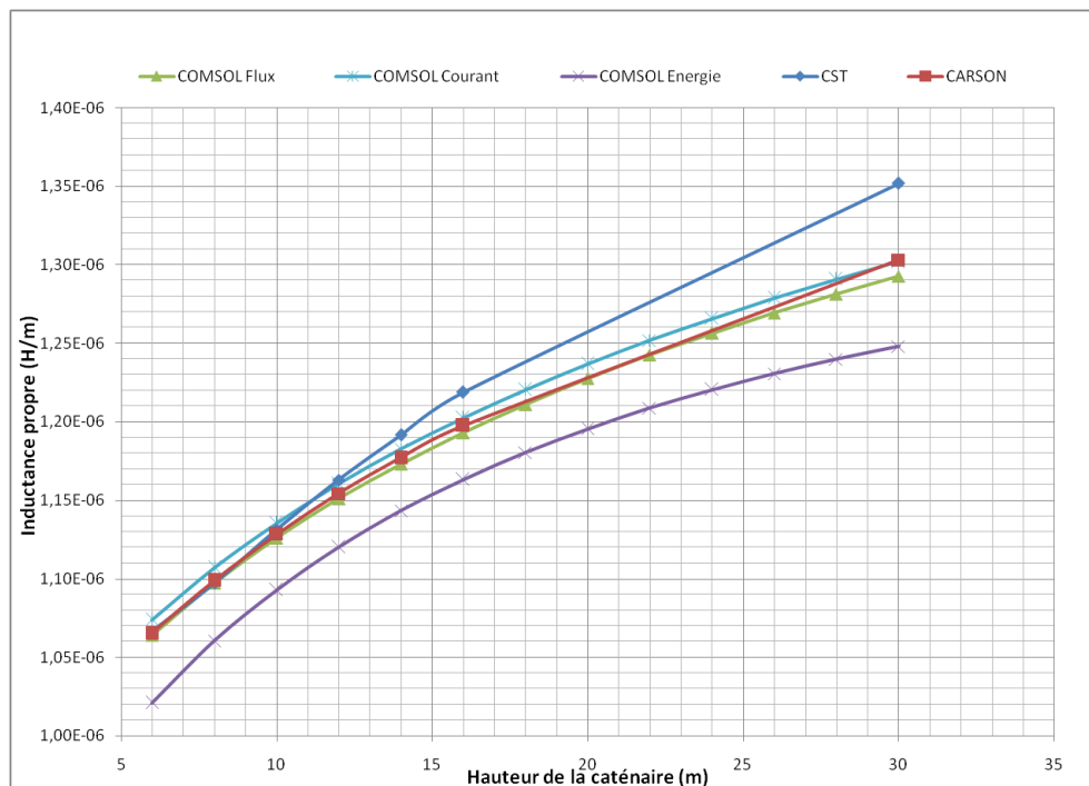
FIGURE 3.2.6 – Inductance propre en fonction de la hauteur de la caténaire.
