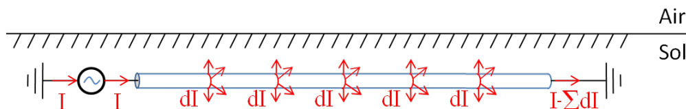
FIGURE 3.2.21 – Injection de courant dans le sol par un conducteur enterré alimenté.
