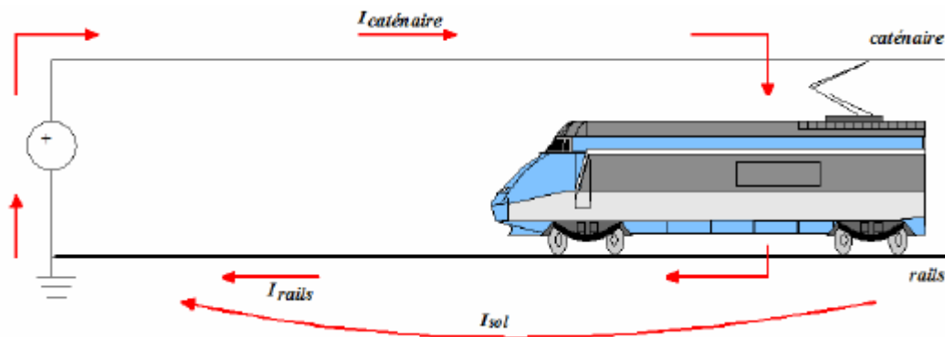
FIGURE 1.1.2 – Schéma simplifié de la boucle du courant d'alimentation.
