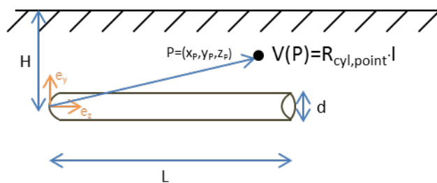
FIGURE 1.2.8 – Couplage entre électrode cylindrique et électrode ponctuelle placée au point P .
